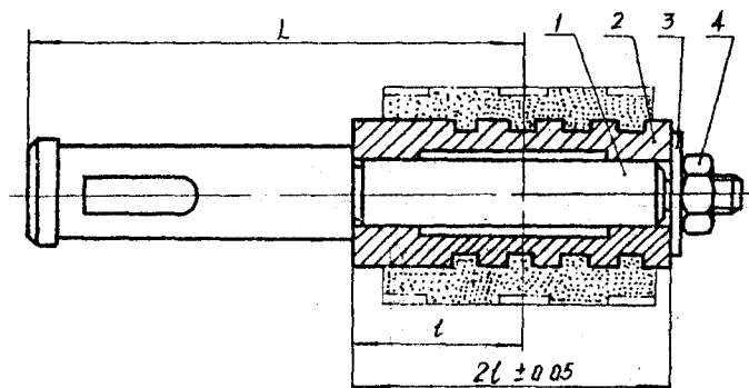
标记示例 l=25 L=100 的标柱样件标高柱 25×100 HB994-89
